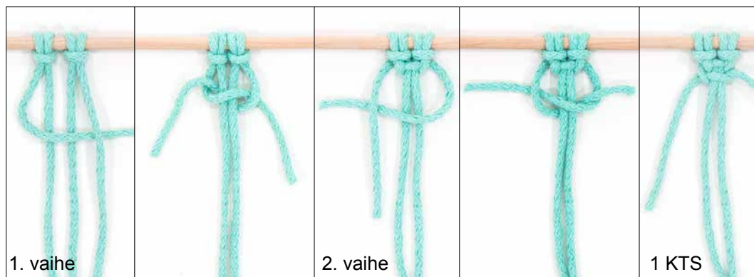
Kuva 3: kaksoistasosolmu
